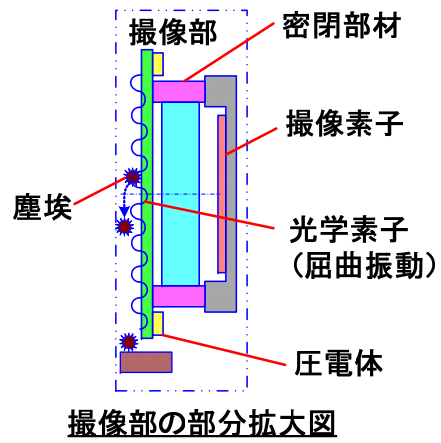
本発明デジタル一眼レフカメラの構造と塵埃
