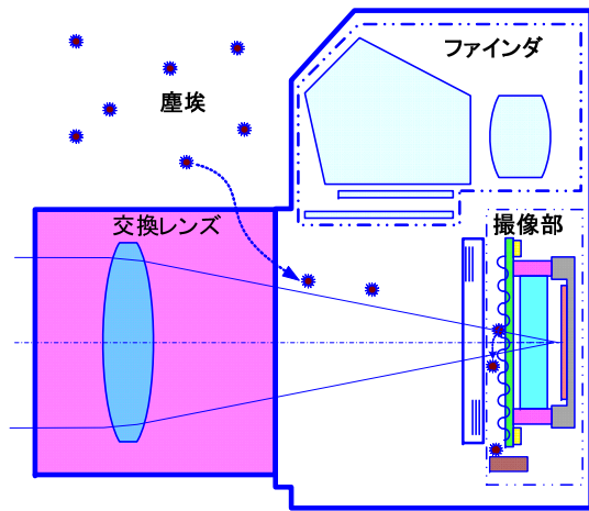
本発明デジタル一眼レフカメラの構造と塵埃
