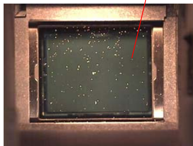
(1) 振動前
